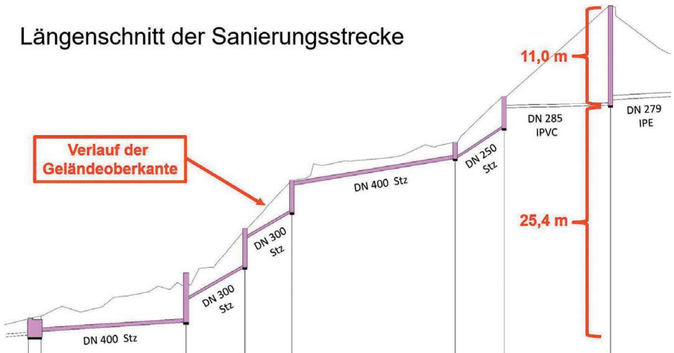
Längenschnitt der Sanierungsstrecke Planung | Grafik: Markus Dohmann
