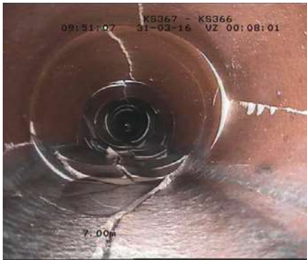
Riss- und Scherbenbildungen sowie massiver Wurzeleinwuchs in den Haltungen | Fotos: Andreas Huber
